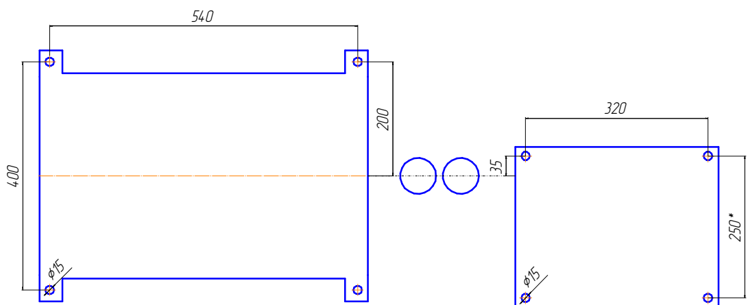
План анкеров
