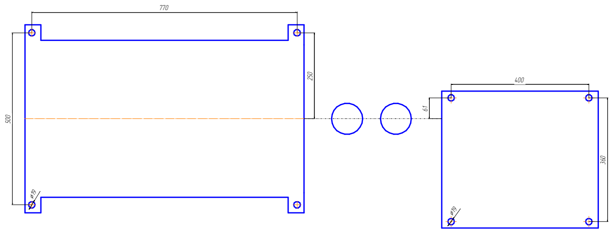
План анкеров
