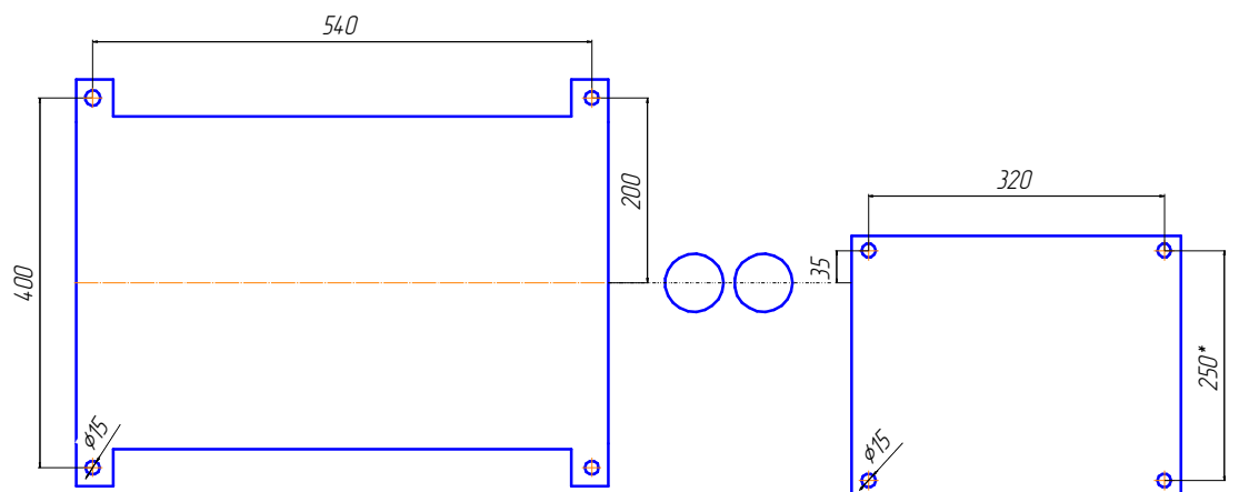
План анкеров
