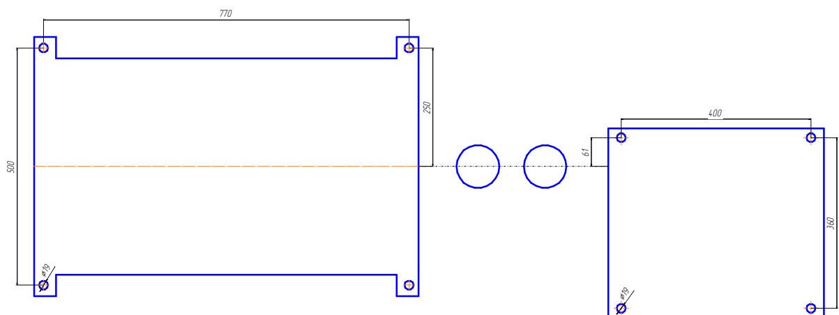
План анкеров
