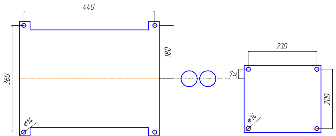
План анкеров
