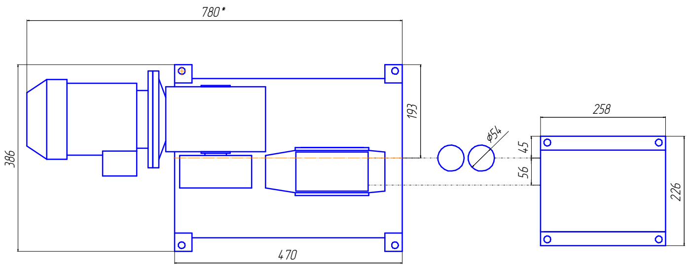
План анкеров
