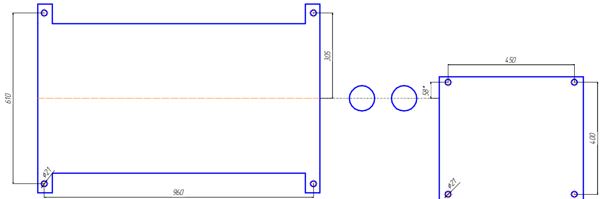
План анкеров
